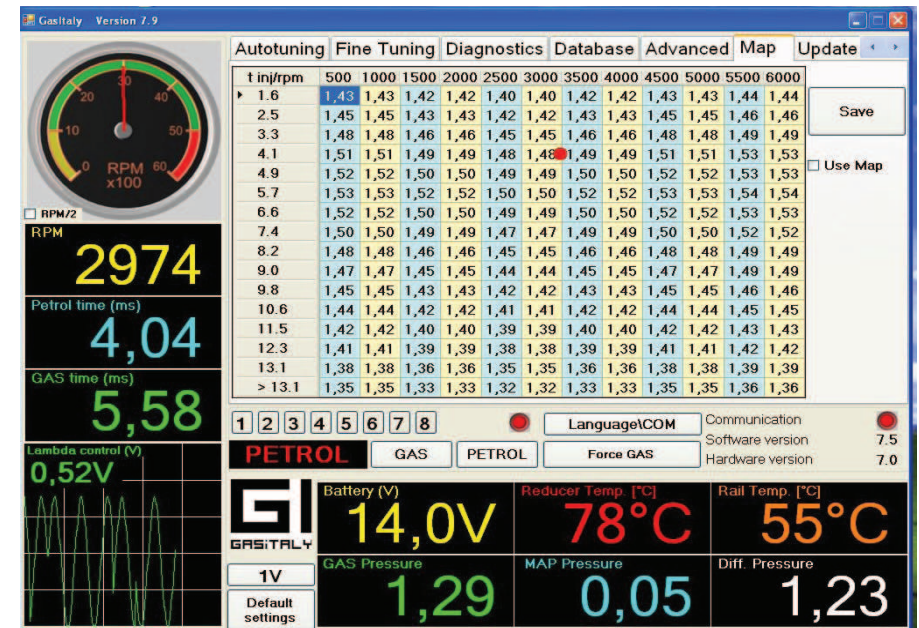
Pic.7 MAP
