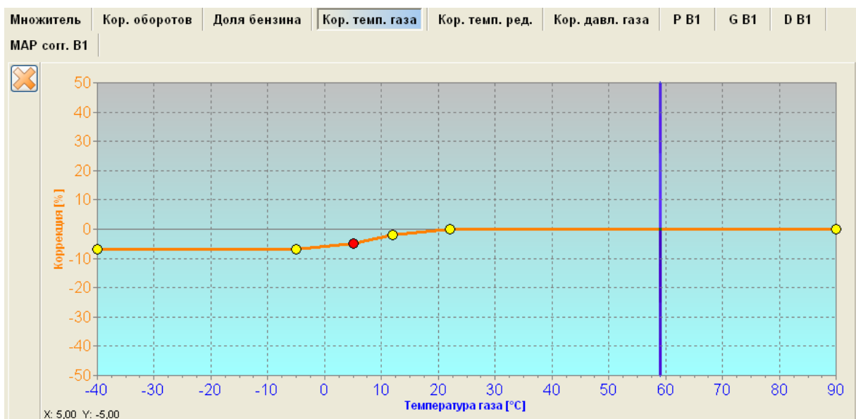
Рисунок 27 Карта «Коррекция температуры газа».
