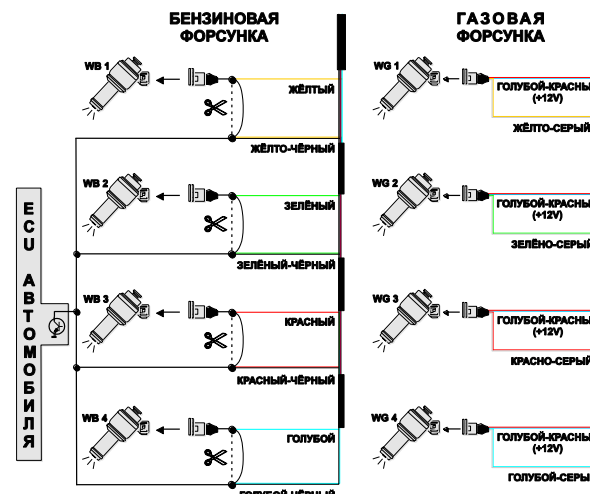
Рисунок 4 Схема подключения к автомобильному оборудованию при управлении «full group».
