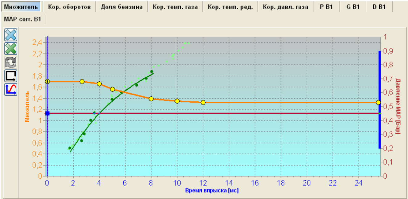
Рисунок 21 Карта множителя. Предлагаемая область «сбора» бензиновой карты.
