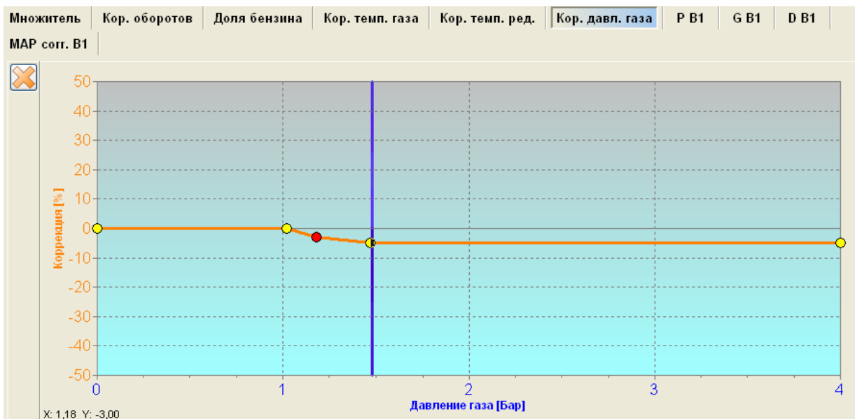
Рисунок 29 Карта «Коррекция давления газа».
