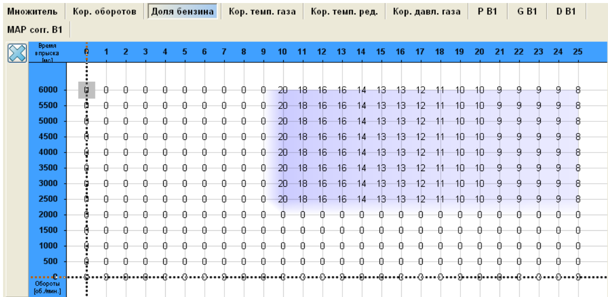
Рисунок 26 Карта доли бензина
