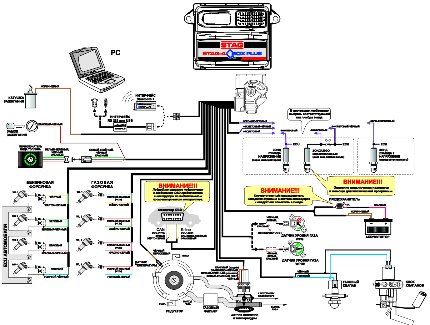
Рисунок 2 Схема подключения STAG-4 Q-BOX PLUS к автомобильному оборудованию.
