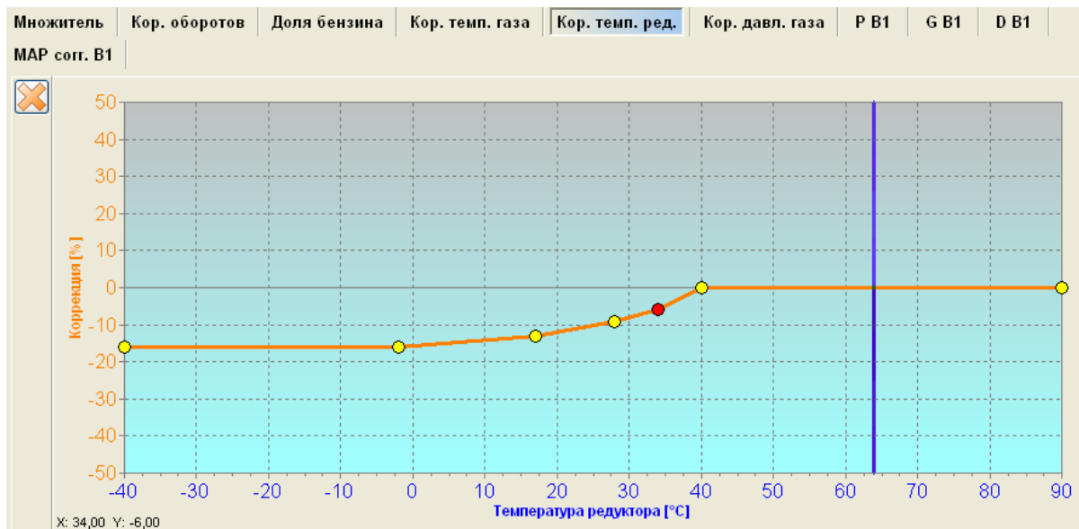
Рисунок 28 Карта «Коррекция температуры редуктора».
