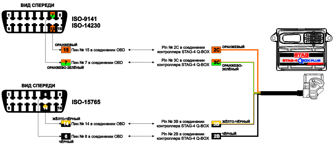
Рисунок 2а Схема подключения STAG-4 QBOX PLUS в разъем OBD.
