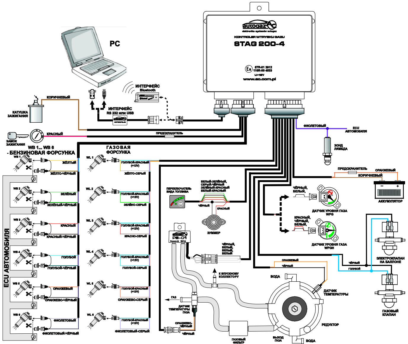
Рис. 1 Схема подключения проводов на автомобиле для STAG-200.
