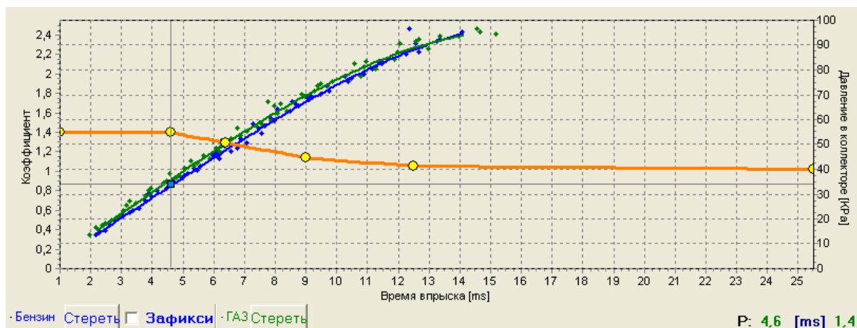
Рис. 16 Карта контроллера
