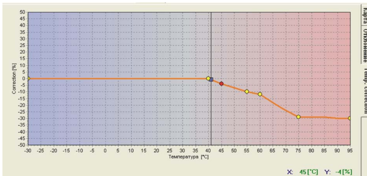
Рис. 20 Вид карты коррекции от температуры газа.
