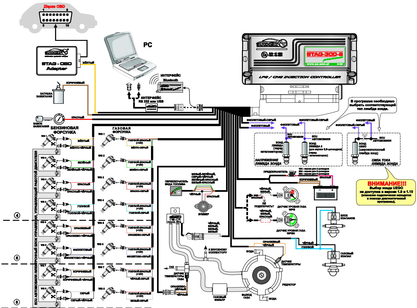
Рис. 4 Схема подключения проводов на автомобиле для STAG-300 Premium.
