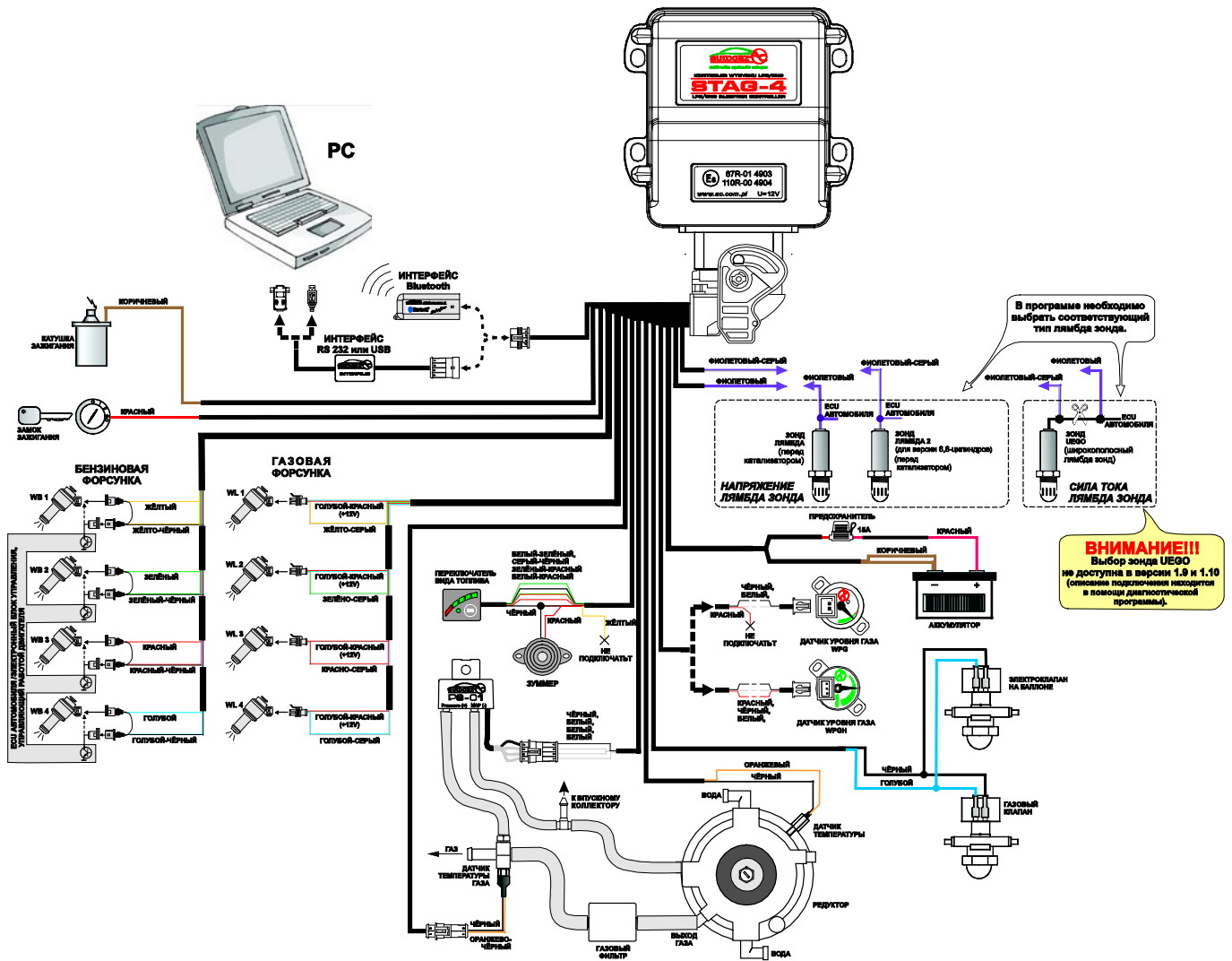
Рис. 2 Схема подключения проводов на автомобиле для STAG-4.
